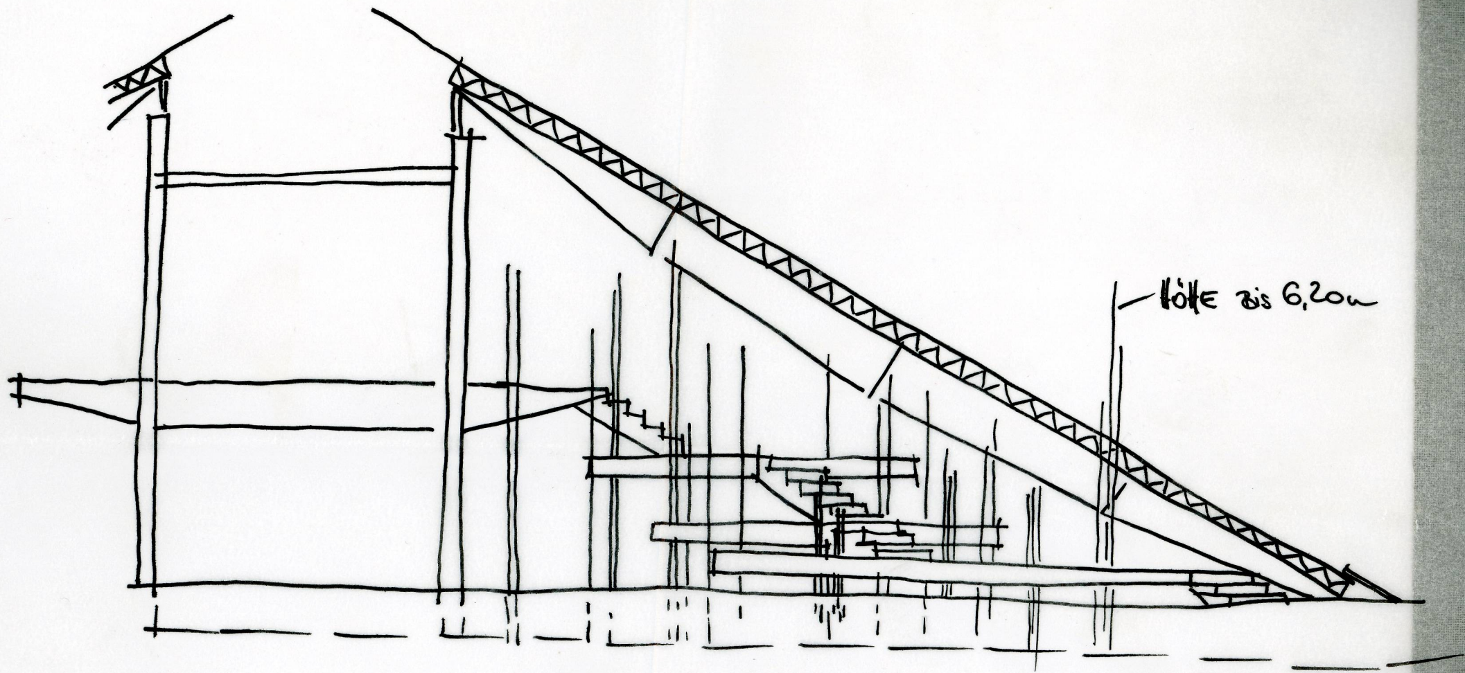
ANSICHT SÜD (VON AVENIDA AUS)
